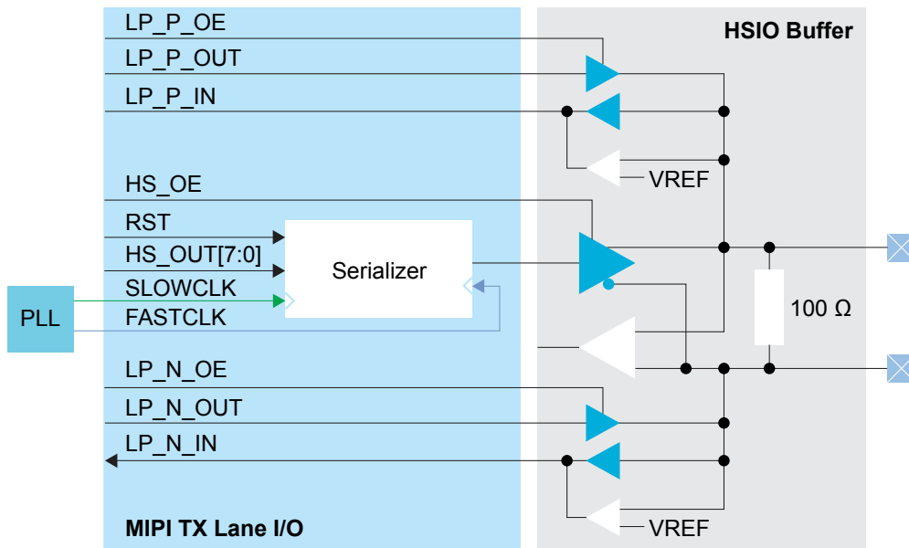
图 31: MIPI TX Lane Block Diagram
