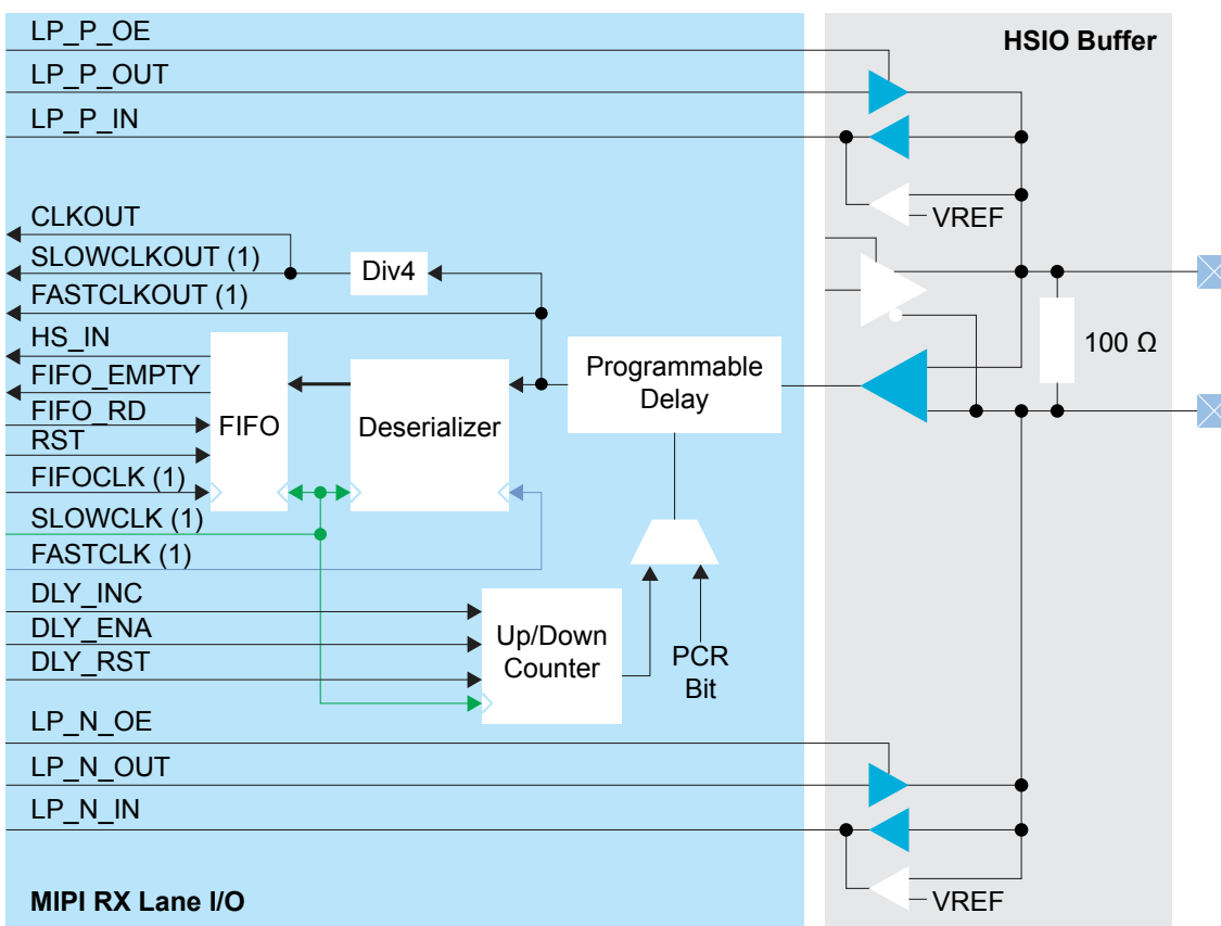
图 29: MIPI RX Lane Block Diagram
