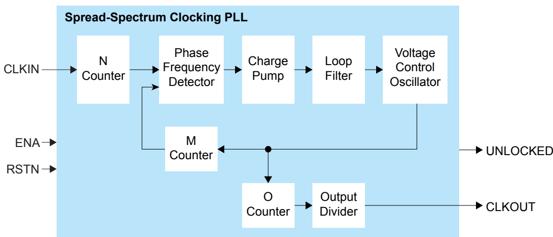
图 42: SSC PLL Block Diagram
