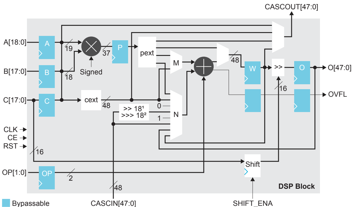
图 5: DSP Block Diagram
