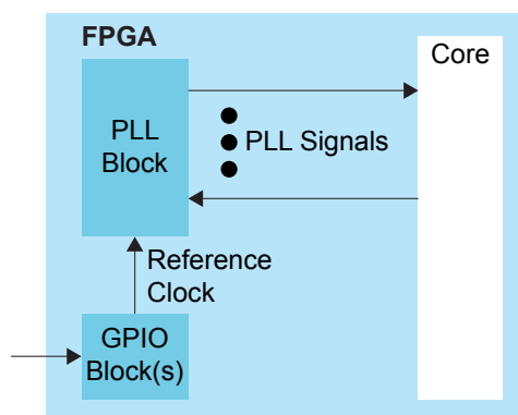
图 43: SSC PLL Interface Block Diagram
