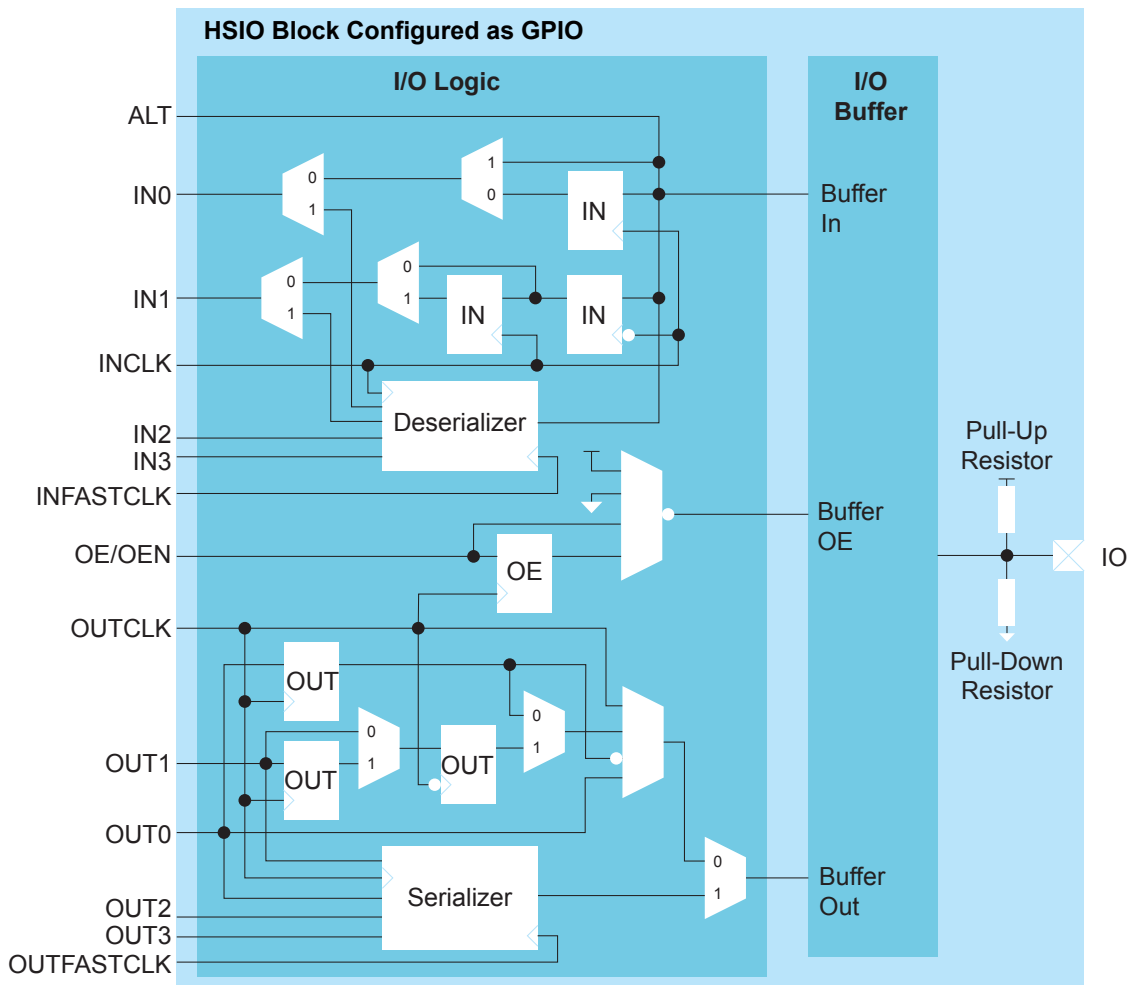
图 20: I/O Interface Block
