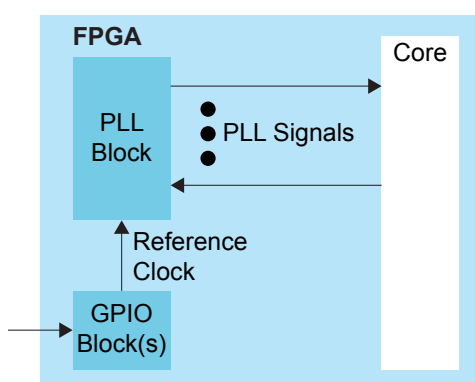
图 43: SSC PLL Interface Block Diagram
